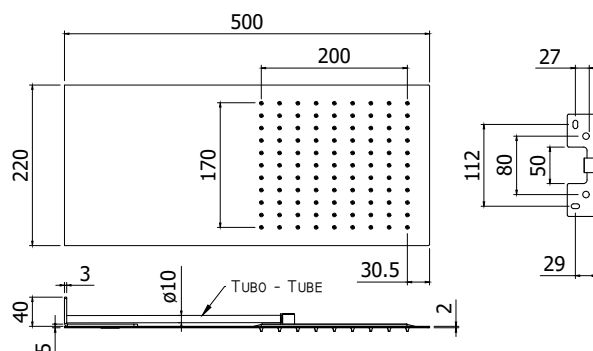
DISEGNO TECNICO
