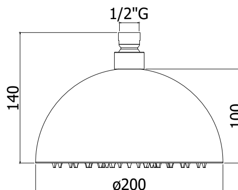
DISEGNO TECNICO
