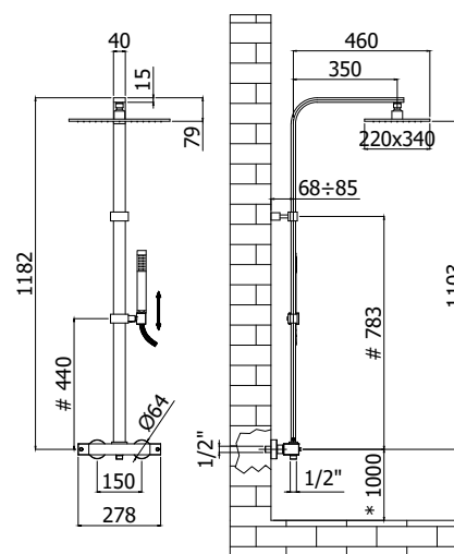
DISEGNO TECNICO
