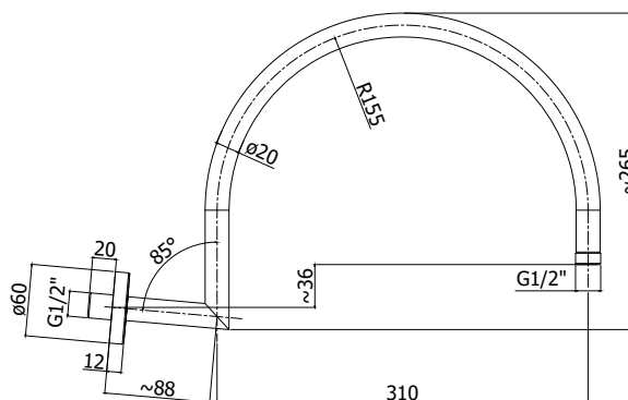
DISEGNO TECNICO
