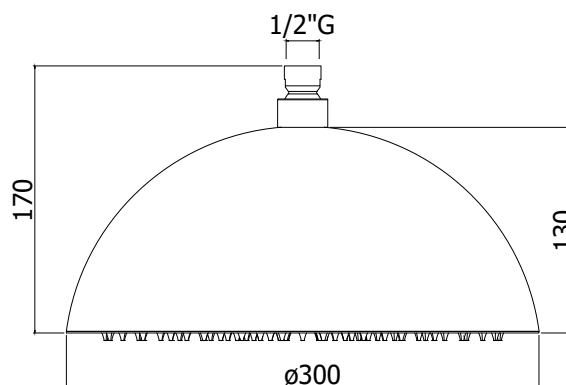
DISEGNO TECNICO
