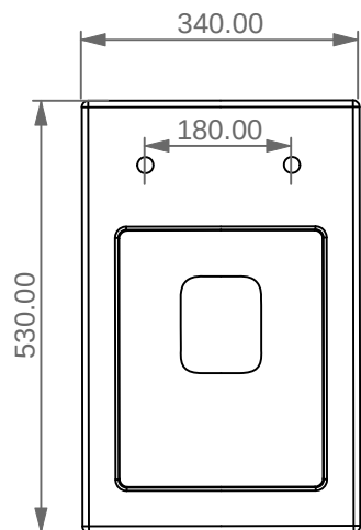
TOP
